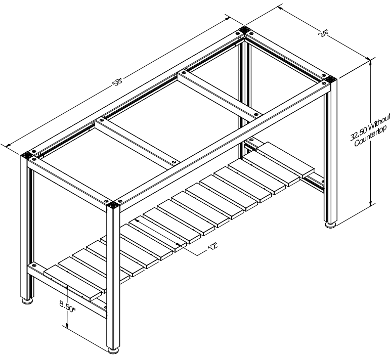
Cosmopolitan Table Dining ADA
